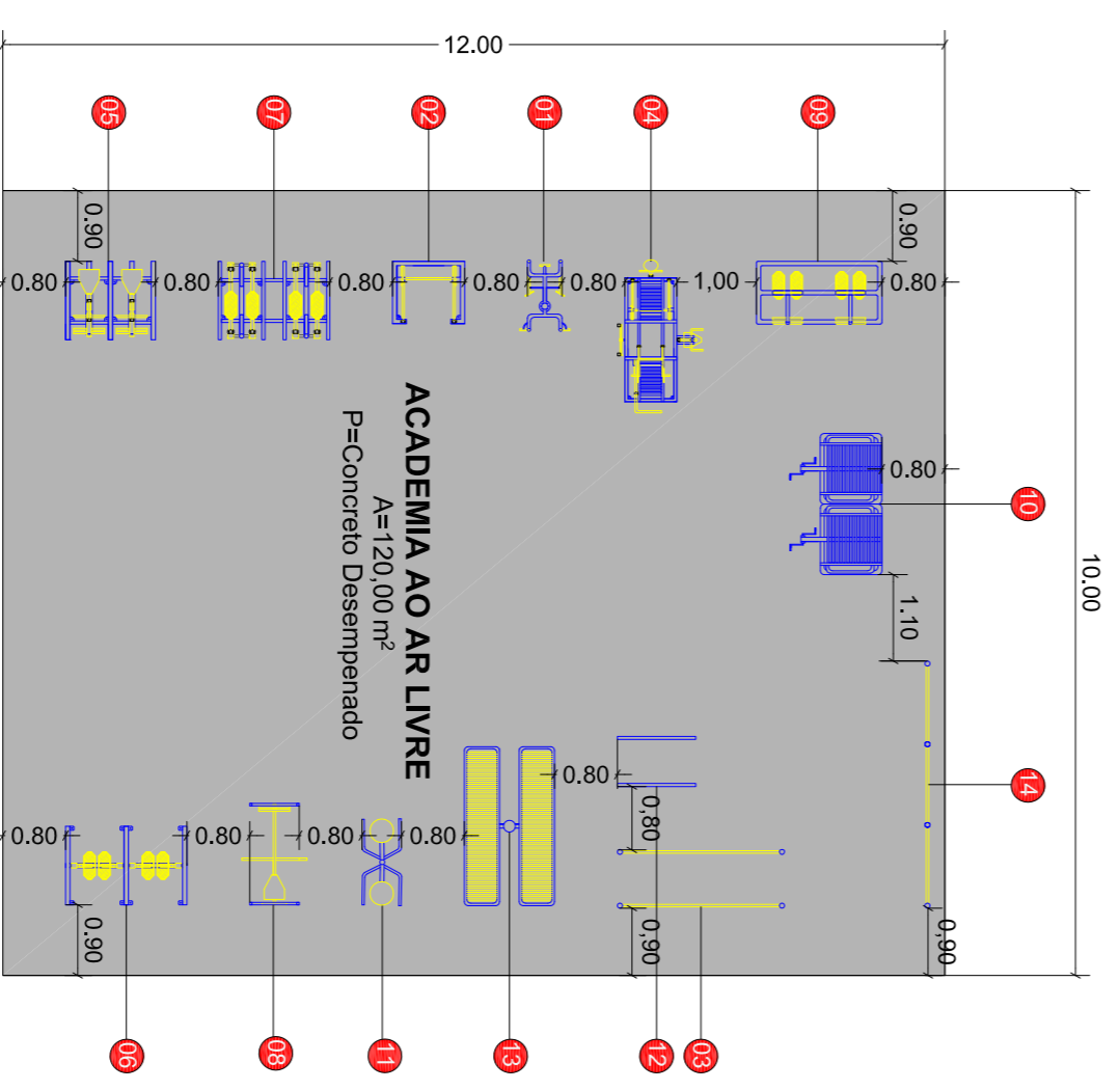
PLANTA BAIXA ÁREA: 120,00m² ESC.: 1/100
