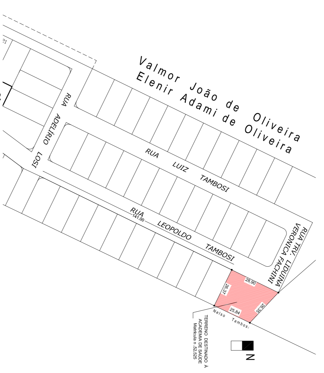
SITUAÇÃO ESC.: 1/1500
