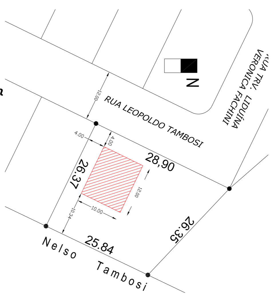
LOCAÇÃO ESC.: 1/500
