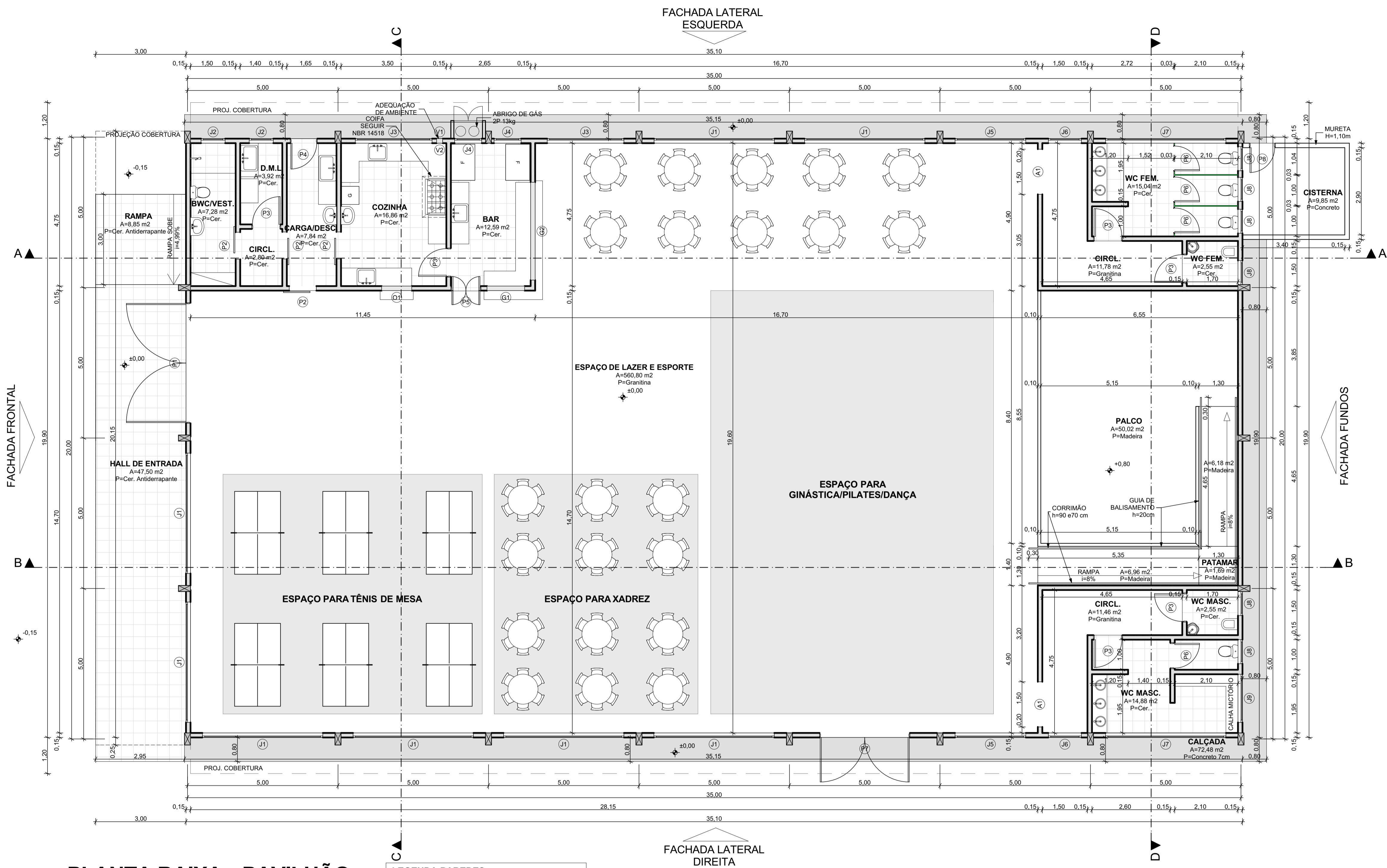
PLANTA BAIXA - PAVILHÃO ÁREA TOTAL: 698,49m 2 ESC.: 1/75
